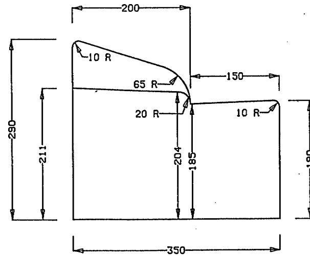
ROLL CURB
